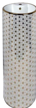
DWSB-3503 (L 400 W 390 H 830mm)
